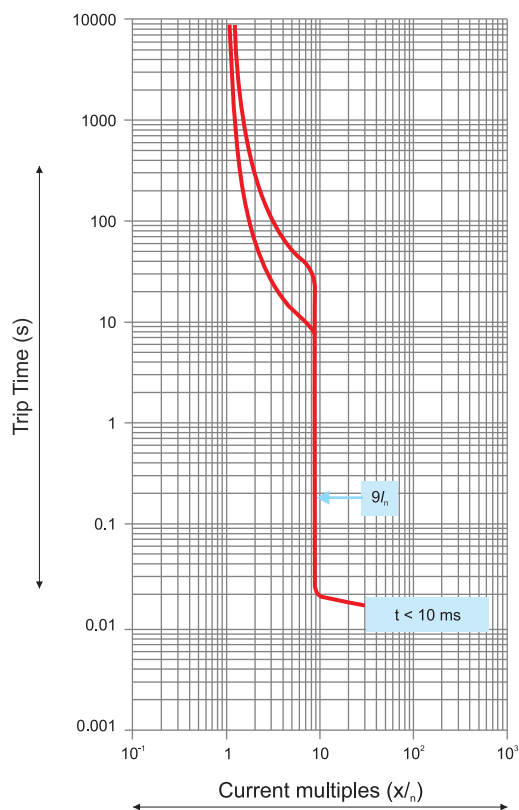
DY250U1 / DU250C / DU250
