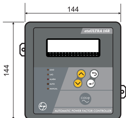
etaULTRA 8R, etaULTRA 16R, etaULTRA 8T+2R, etaULTRA 14T+2R & etaULTRA 8T+8R
