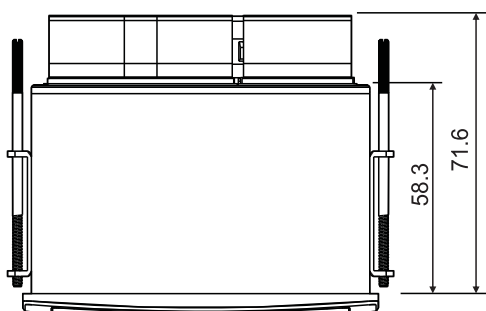
etaULTRA 8R, etaULTRA 16R, etaULTRA 8T+2R, etaULTRA 14T+2R & etaULTRA 8T+8R
