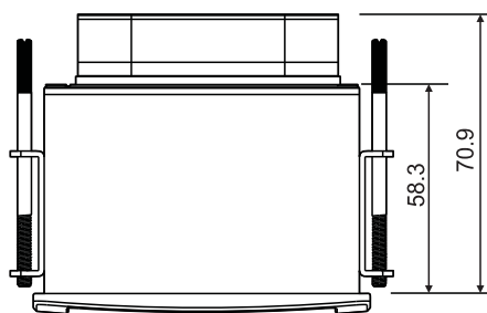
etaSMART 4R, etaSMART 6R, etaSMART 8R and etaSMART 6T
