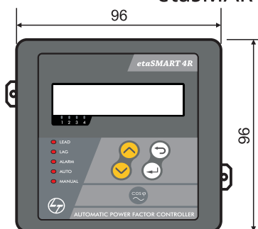
etaSMART 4R, etaSMART 6R, etaSMART 8R and etaSMART 6T
