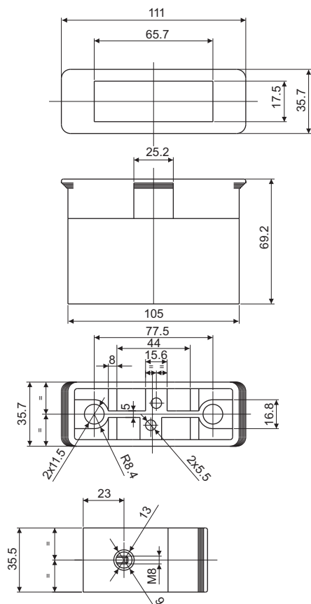
HK 63
