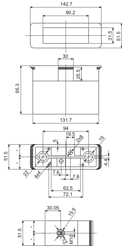
HK 125
