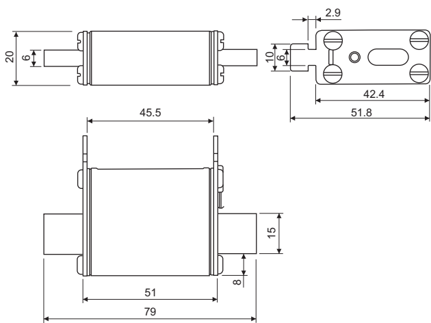
Size 000
