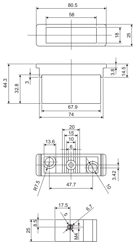
HD 20 / HD 32
